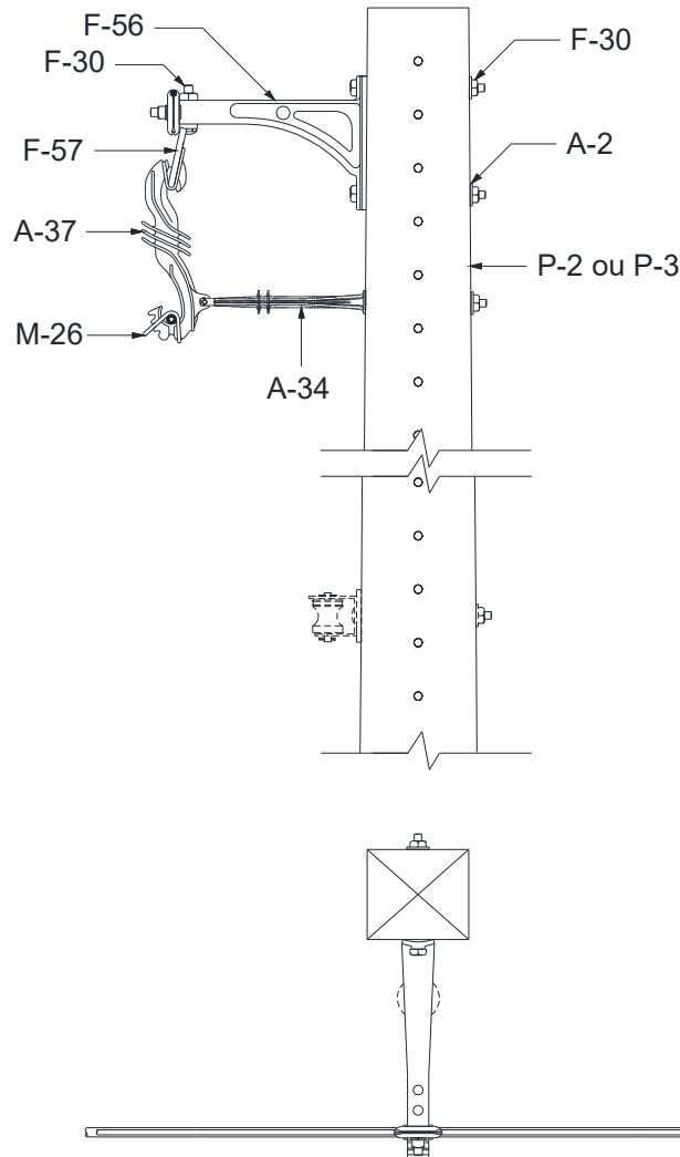
Figura 20 – Estrutura CU1A – Poste de seção DT ou de madeira
